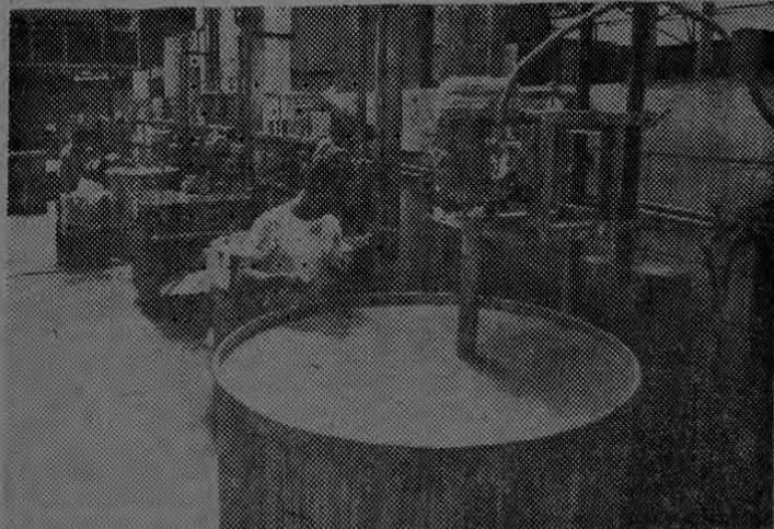
ZONA DE MEZCLA DE PINTURAS— Estos tanques están provistos de un eje en posición vertical que remueve a alta velocidad la PASTA BASICA que se procesa previamente en el DISPENSADOR. A esta pasta se agregan los colorantes, solventes y secantes, y se le controla su densidad y viscosidad. Una vez terminada esta operación la pintura queda preparada para el envase.
